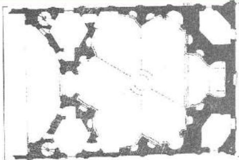
ش ۳ - پلان کلیسای سان ایوو، ایزوگورینی، ایتالیا.
