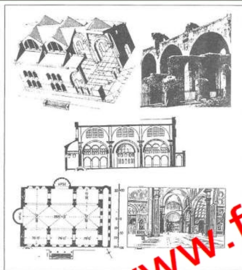
ش ۶۰ - تصویر، پرسپکتیو، نما، مقطع، پرسپکتیو داخلی و پلان باسیلیکا کانسانتین در روم.
