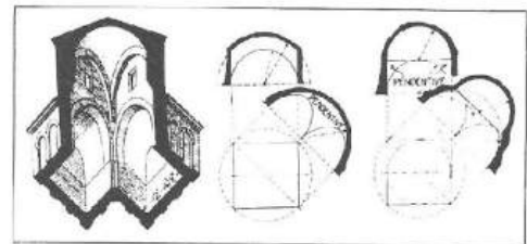
ش ۱۰ - نحوه جایی از نحوه ساخت کردن بناهای بیزانسی.
