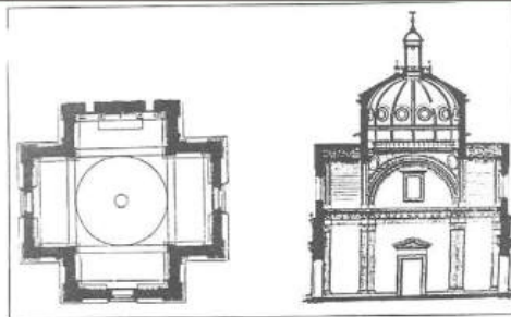
ش ۱۰۲ - پلان و مقطع کلیسای سانتا ماریا ده کالترری ، وینسنگو .
