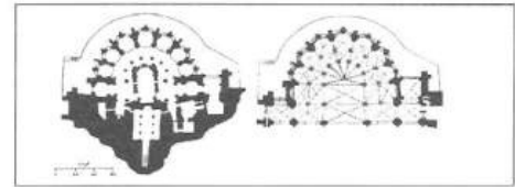
ش ۱ - پلان نمازخانه کلیسای نوتردام، پاریس.
