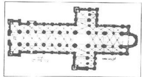
ش ۱۱ - پلان کلیسای دورم.
