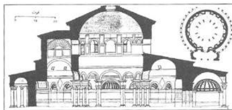
ش ۴ - پلان و مقطع کلیسای سائتاکونستانتینا.
