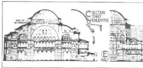
ش ۶ - مقطع و بیسی از مقطع کلیسای ایاصوفیه ، استانبول .
