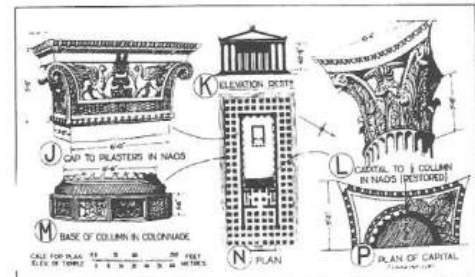
ش ۱۴ - پلان، نما و جزئیات ستون های معبد آپولون در شهر دیدوما.
