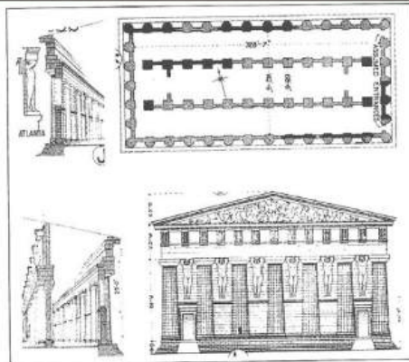
ش ۷ - پلان، نما و مقطع معبد ژنوس، اسیلیا.
