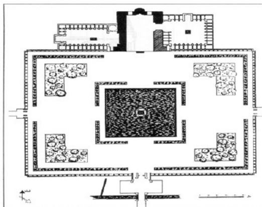
نقشه ایوان بزرگ ارگ با مسجد جامع علیشاه و ساختمان های مجاور آن، ( اردک، راز )
