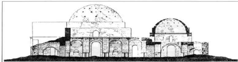
کاخ سروستان، برش از اتاق کنگد دار کوچک (نسخه از مسعودی، سنی، ایران)
