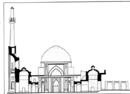
یزد مسجد جامع، برش و نما (زیمه‌ن)
