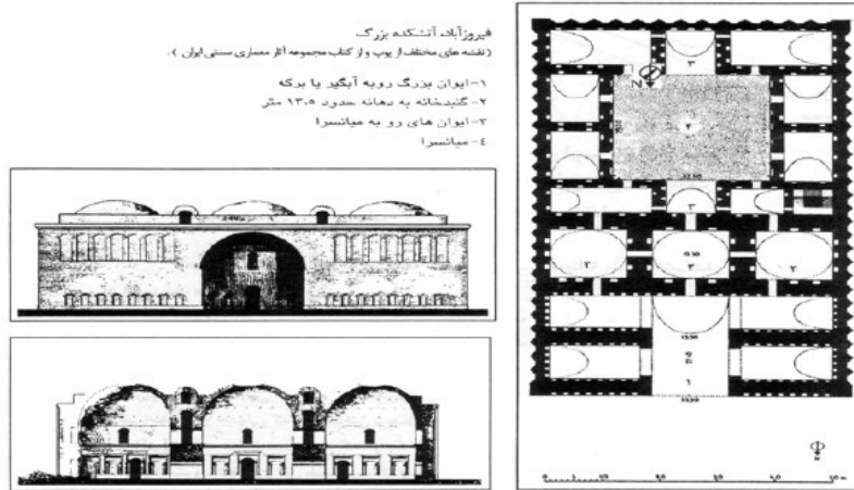
آتشکده فیروزآباد نمای اصلی. آتشکده فیروزآباد، برش از سه کنیشتانه.
