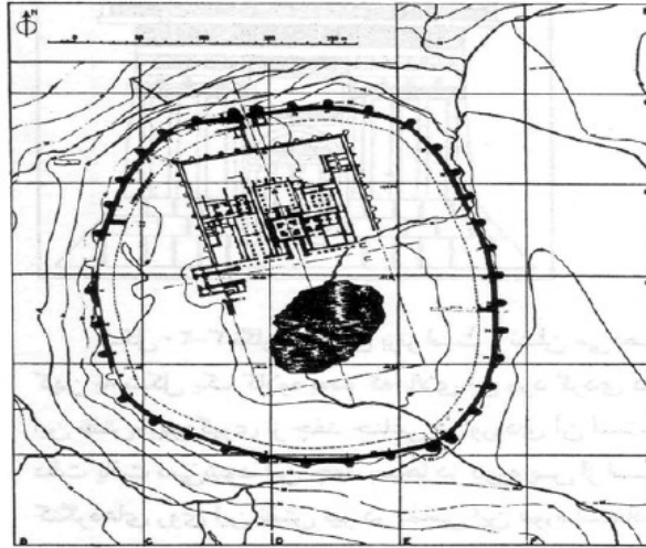
نقشه مجموعه تخت سلیمان شامل آبگیر یا برکه، دیوار دور و ساخته‌های گوناگون (از بوب).
