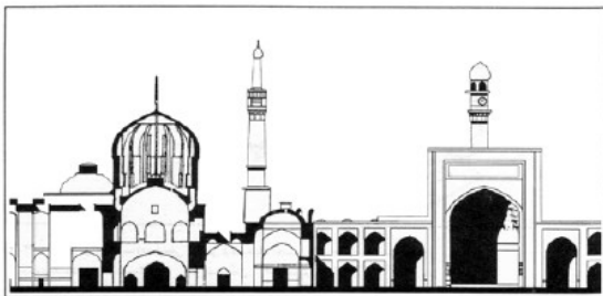
مشاهد برش از گنبدخانه بازگه (در محفل)
